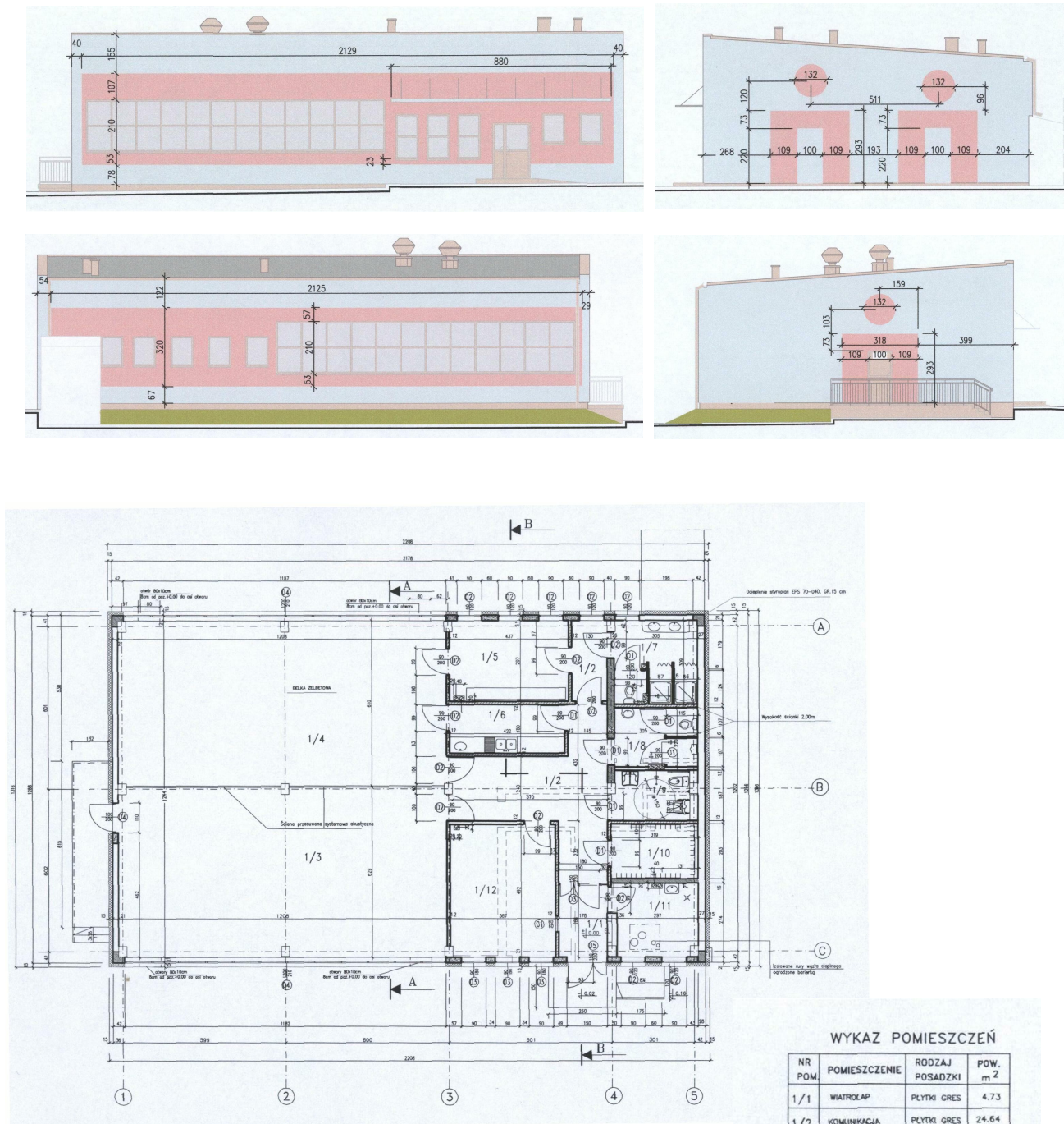
Rys. 10 Widok elewacji oraz rzut parteru budynku wymiennikowni po przebudowie i adaptacji na świetlicę osiedlową
