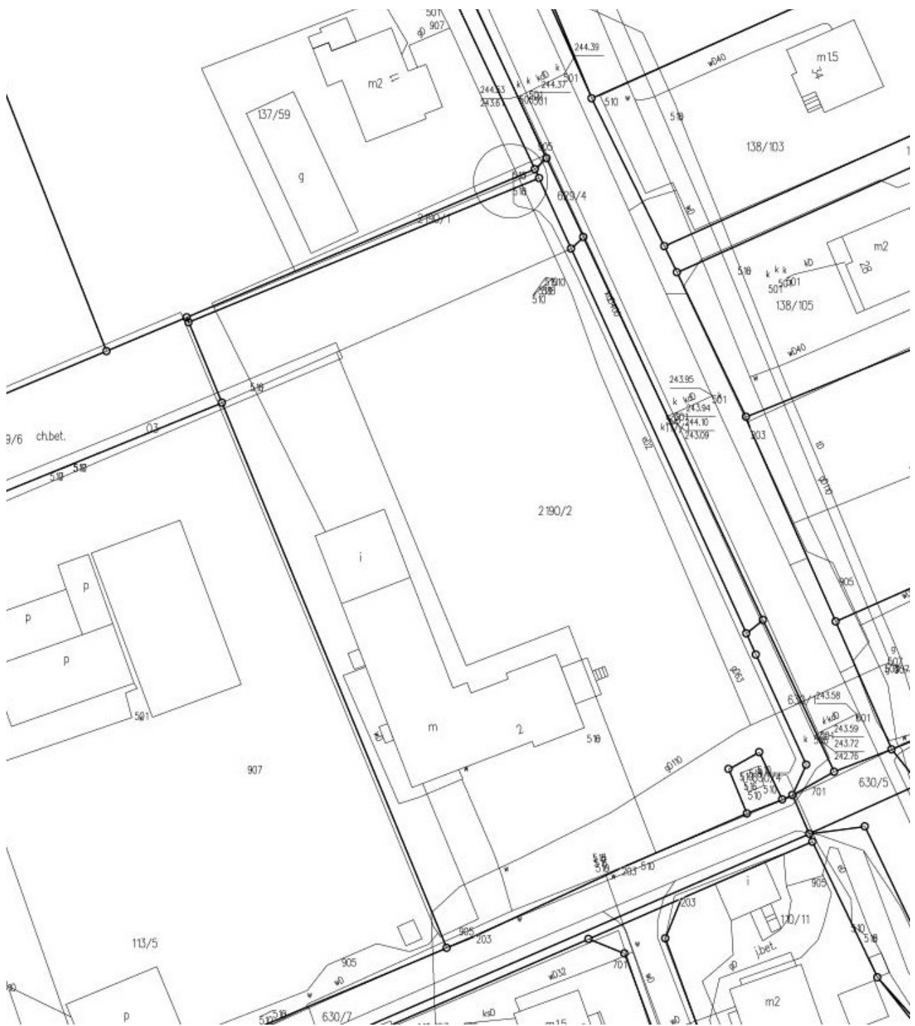
Mapa zasadnicza - wyrys
