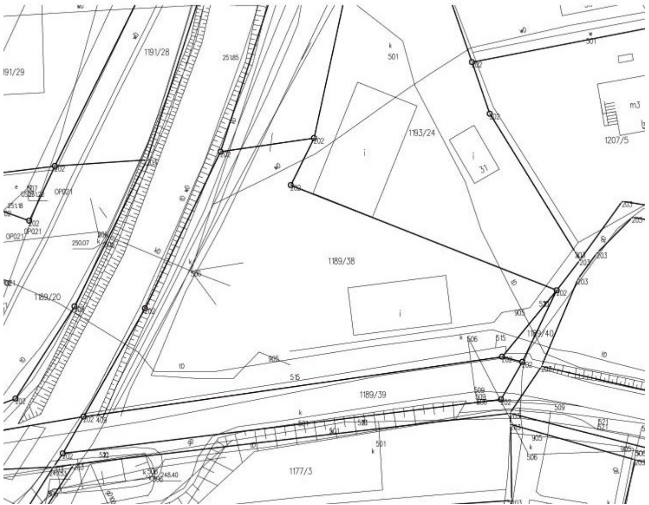
Mapa zasadnicza - wyrys
